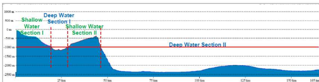
Figura 7.1 - Profundidade (batimetria) para instalação do Ramal de ligação de São Miguel – Açores do cabo do Sistema NUVEM: BU1 –S1.1 (BMH)
