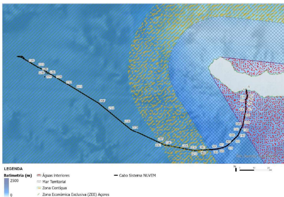
Figura 7.3 – Batimetria GEBCO - Ramal de ligação de São Miguel – Açores do cabo do Sistema NUVEM: BU1 – S1.1 (BMH) (Fonte: Geoportal do Mar Português)
